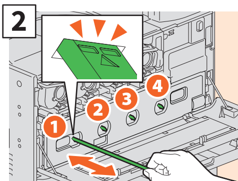
Dra ut rengöraren tills märket syns, och sätt sedan tillbaka den. Upprepa 3 gånger för varje färg.
