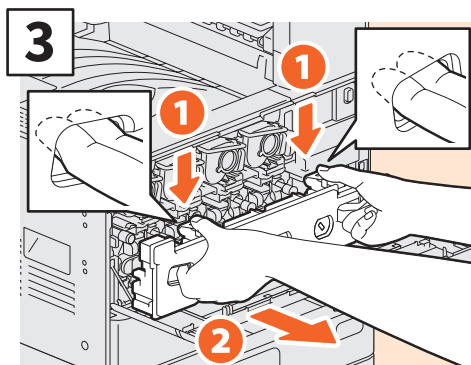
Sätt in fingrarna i resttonerbehållarens främre skåror och ta ut den mot dig samtidigt som du trycker ned övre spärren. Rengör sedan LED-skrivarhuvudena eller slit glaset. Läs följande för anvisningar om hur du rengör LED-skrivarhuvudena eller slit glaset:
